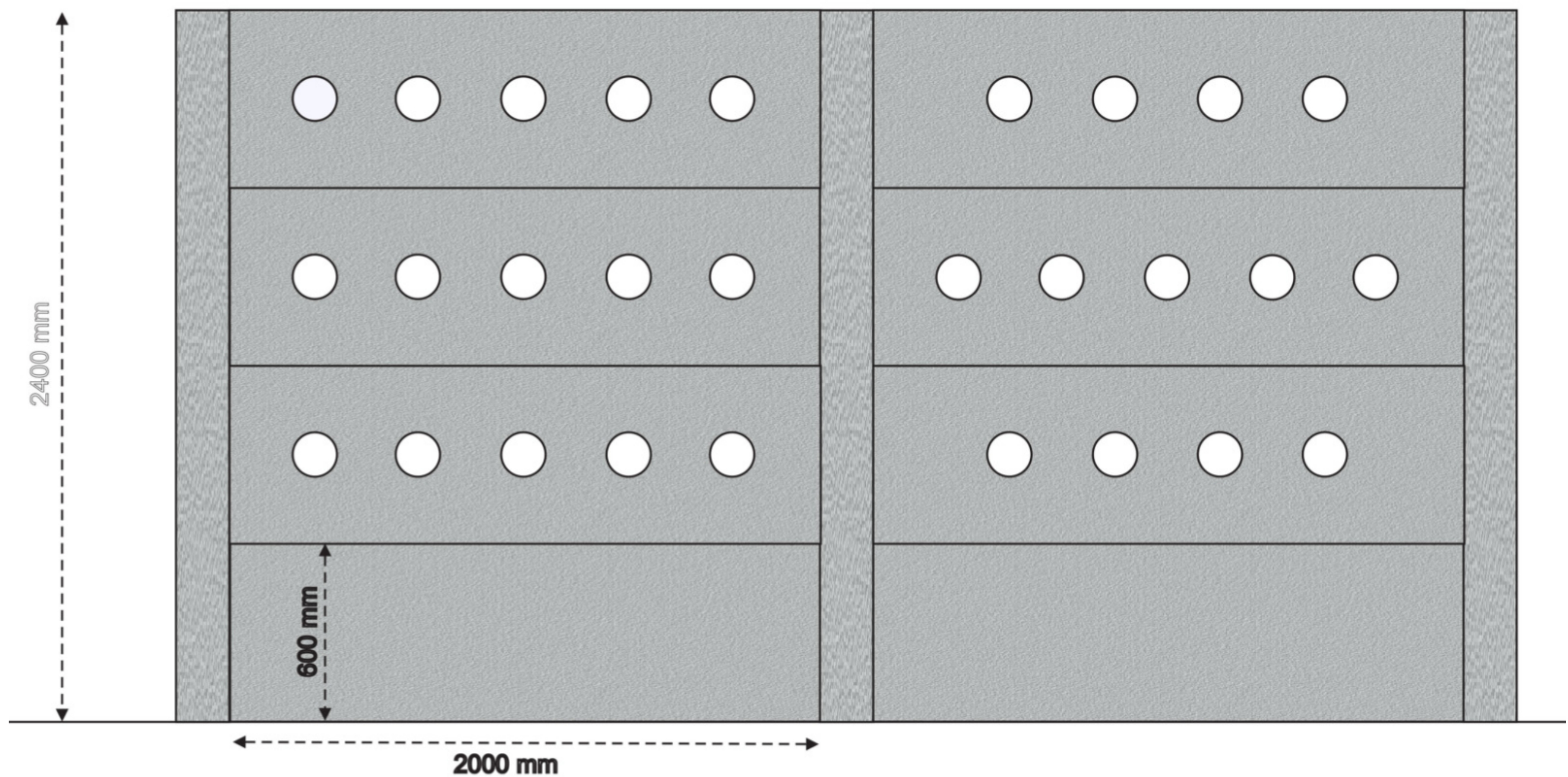
Hình 1: Tường rào lắp ghép mẫu 1
