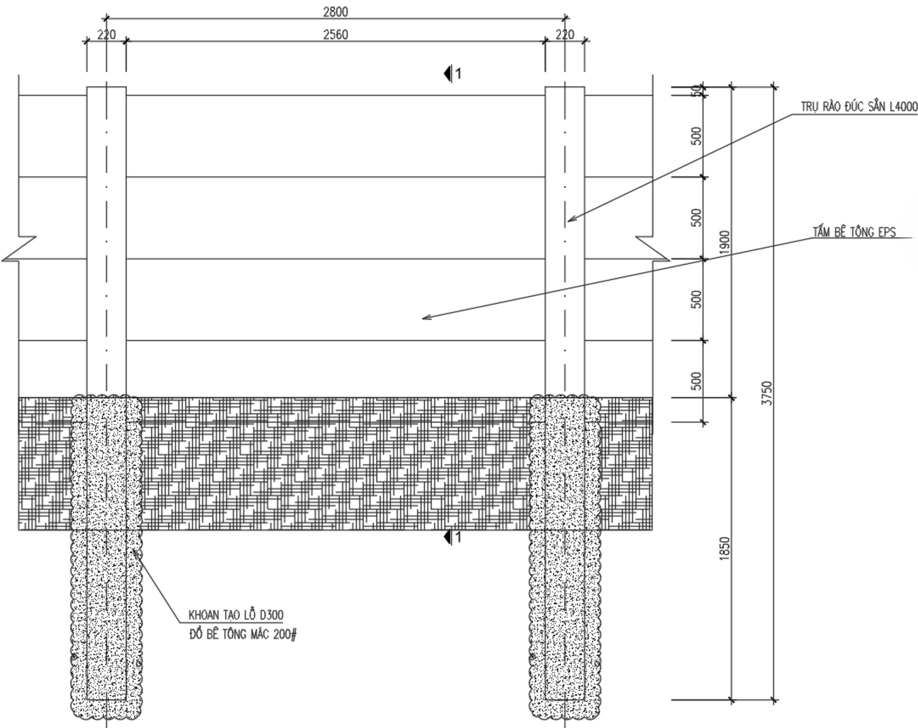
MẶT ĐỨNG ĐOẠN TƯỜNG RÀO LOẠI 3
