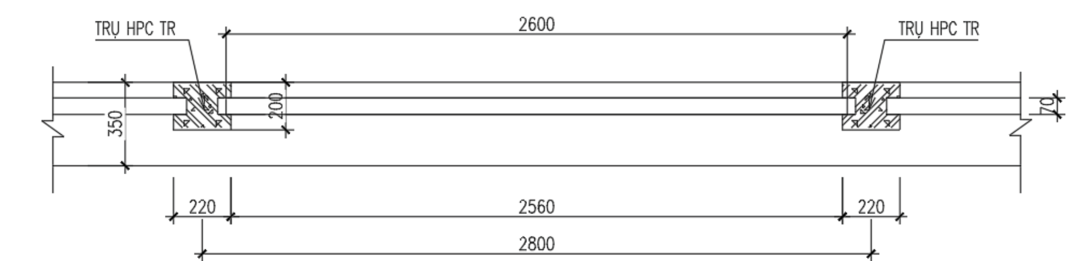
MẶT BẰNG ĐOẠN TƯỜNG RÀO LOẠI 1
