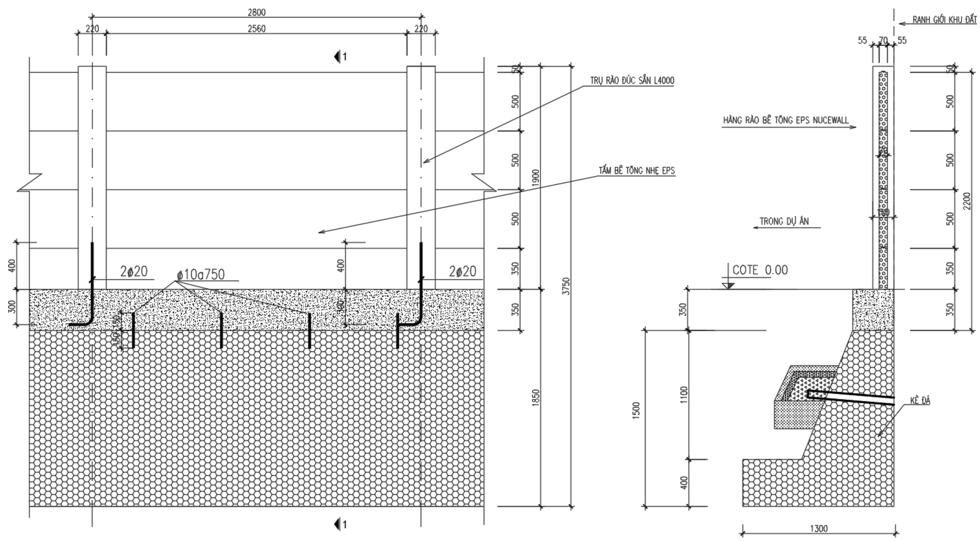
MẶT ĐỨNG ĐOẠN TƯỜNG RÀO LOẠI 1
