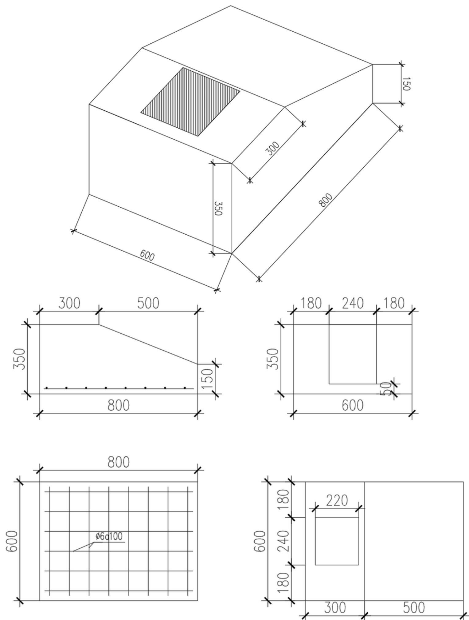
CHI TIẾT CẤU TẠO MÔNG ĐÚC SẴN Ghi chú: Bê tông cốt thép móng - cột #250.
