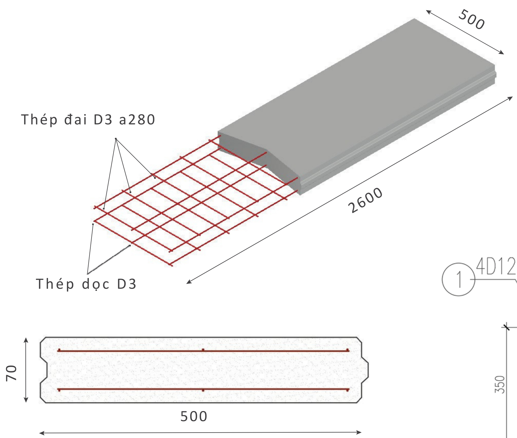
MẶT CẮT NGANG TẤM BÊ TÔNG NHẹ EPS
