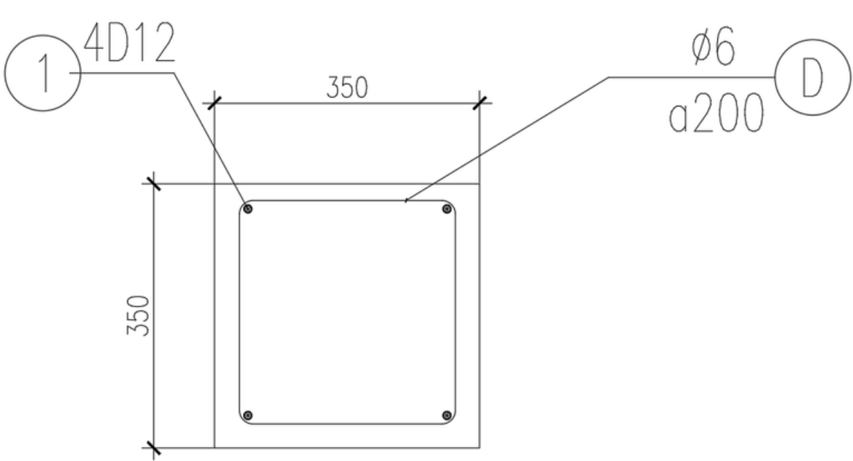
CẤU TẠO GIẺNG KỀ ĐÁ MẶT CẮT 3 - 3 Ghi chú: Bê tông cốt thép giẻng - cột #250.
