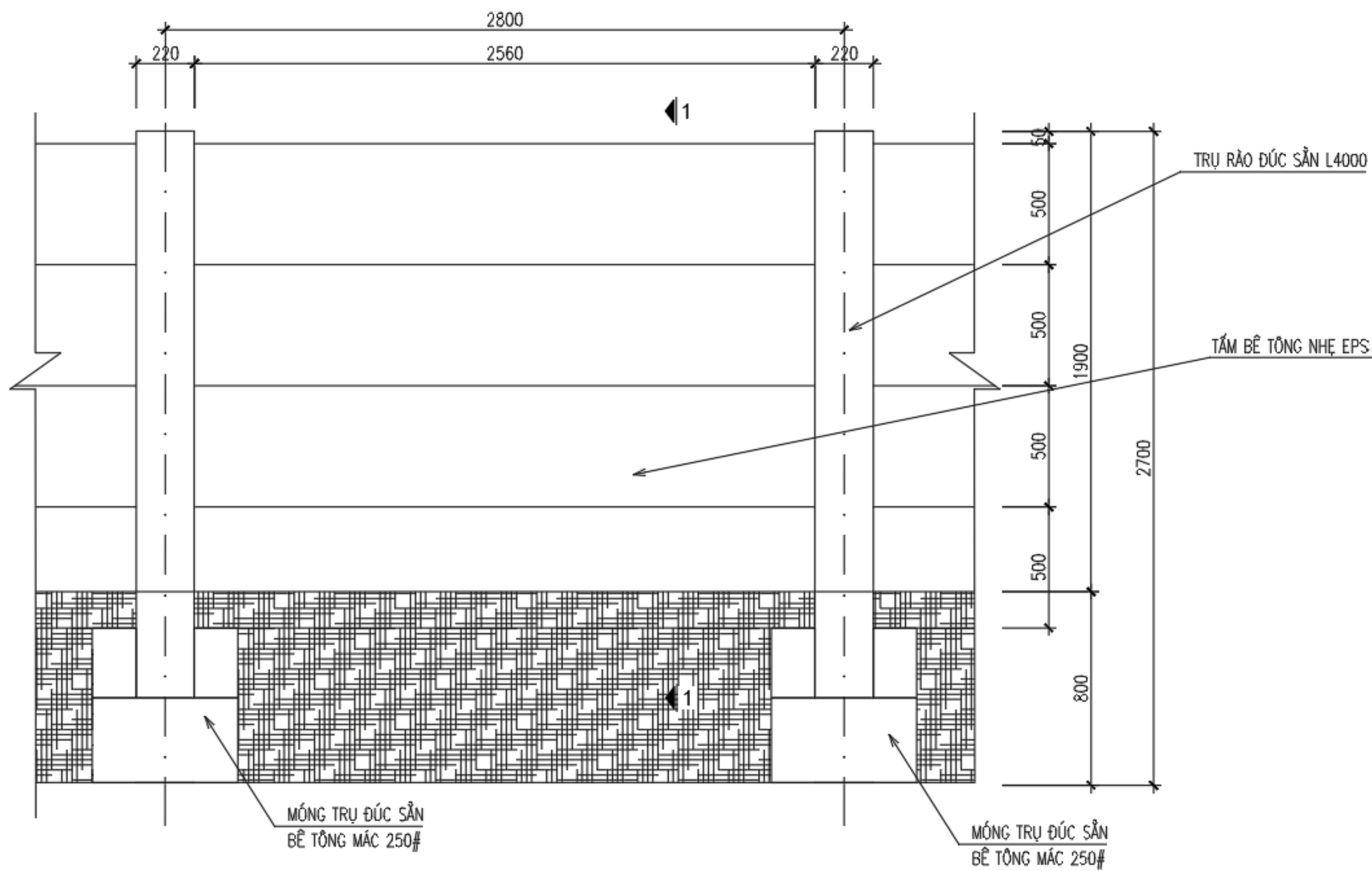
MẶT ĐỨNG ĐOẠN TƯỜNG RÀO LOẠI 2
