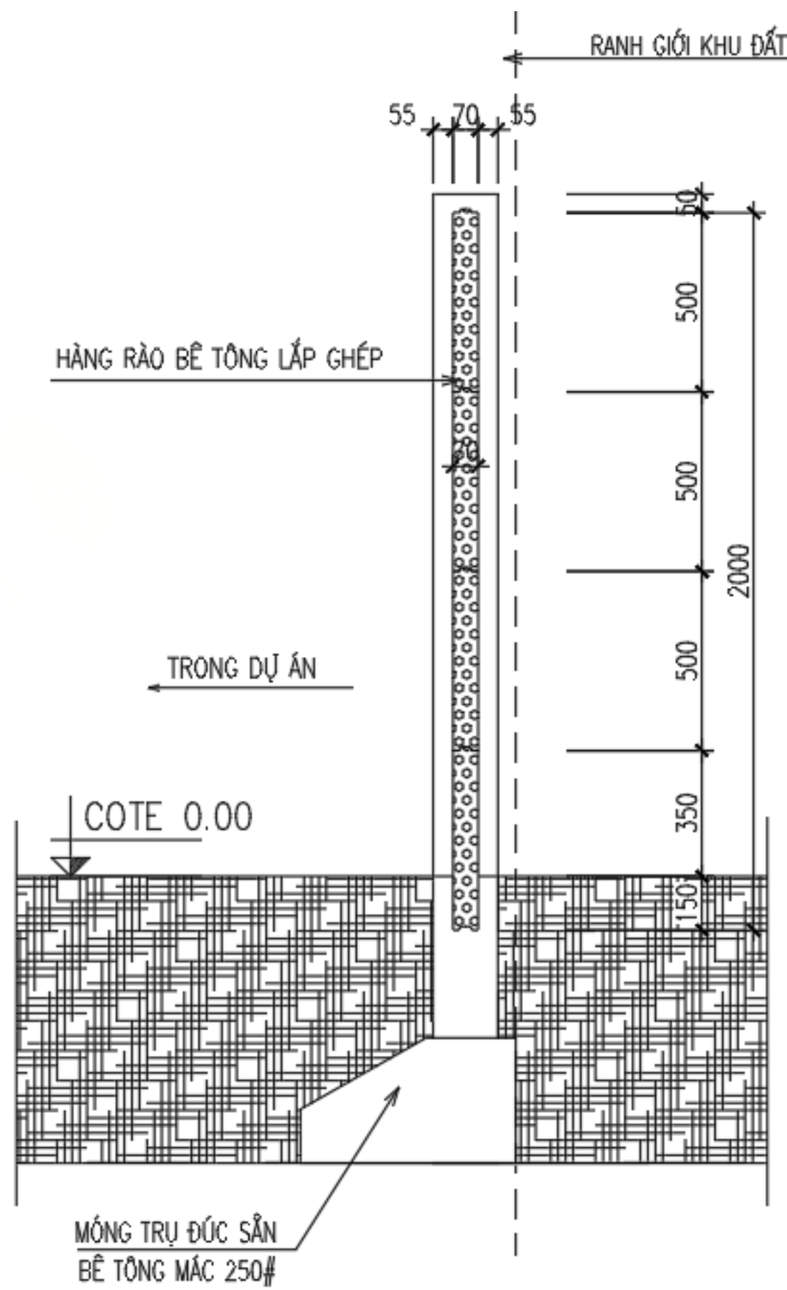
MẶT CẮT 1 - 1
