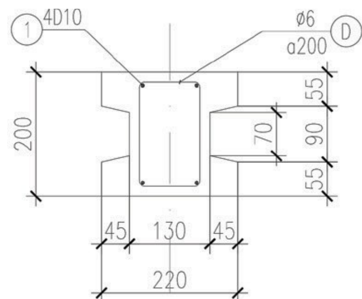
MẶT CẮT 2 - 2
