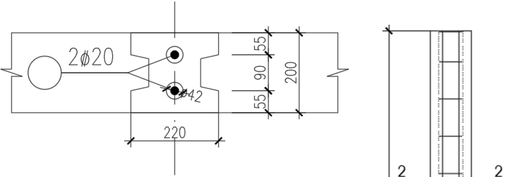
ĐỊNH VỊ THÉP CHỜ LIÊN KẾT CỘT
