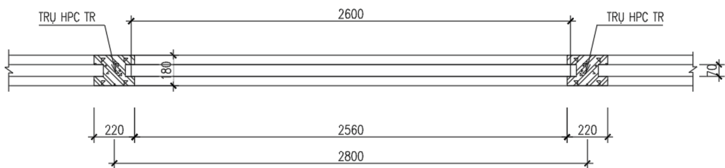
MẶT BẰNG ĐOẠN TƯỜNG RÀO LOẠI 2
