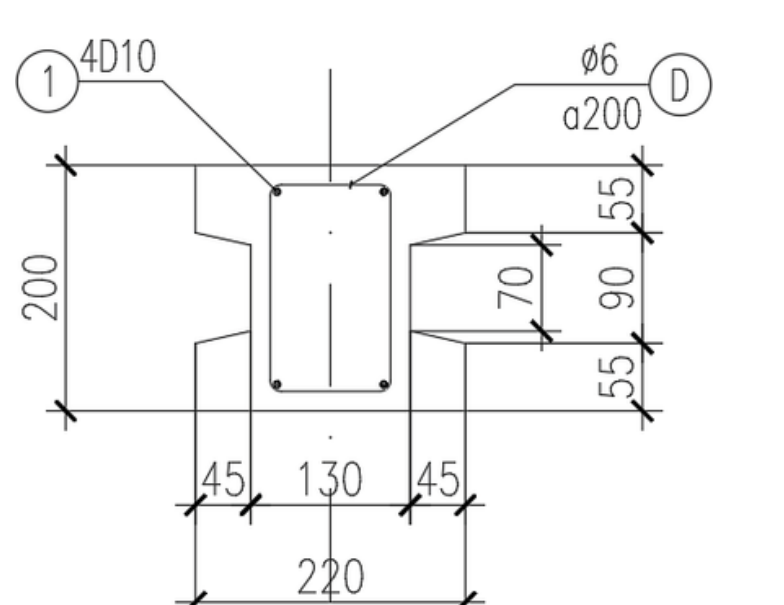
MẶT CẮT 2 - 2
