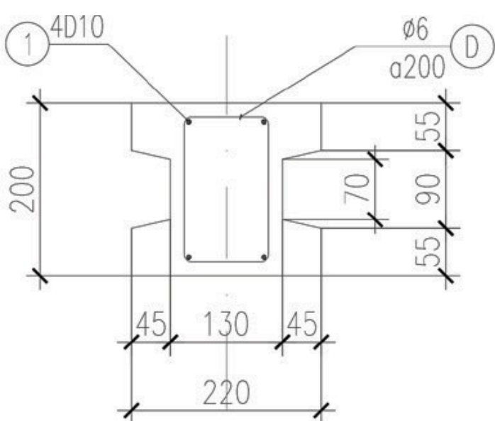
MẶT CẮT 2 - 2 Ghi chú: Bê tông cốt thép cột #250.
