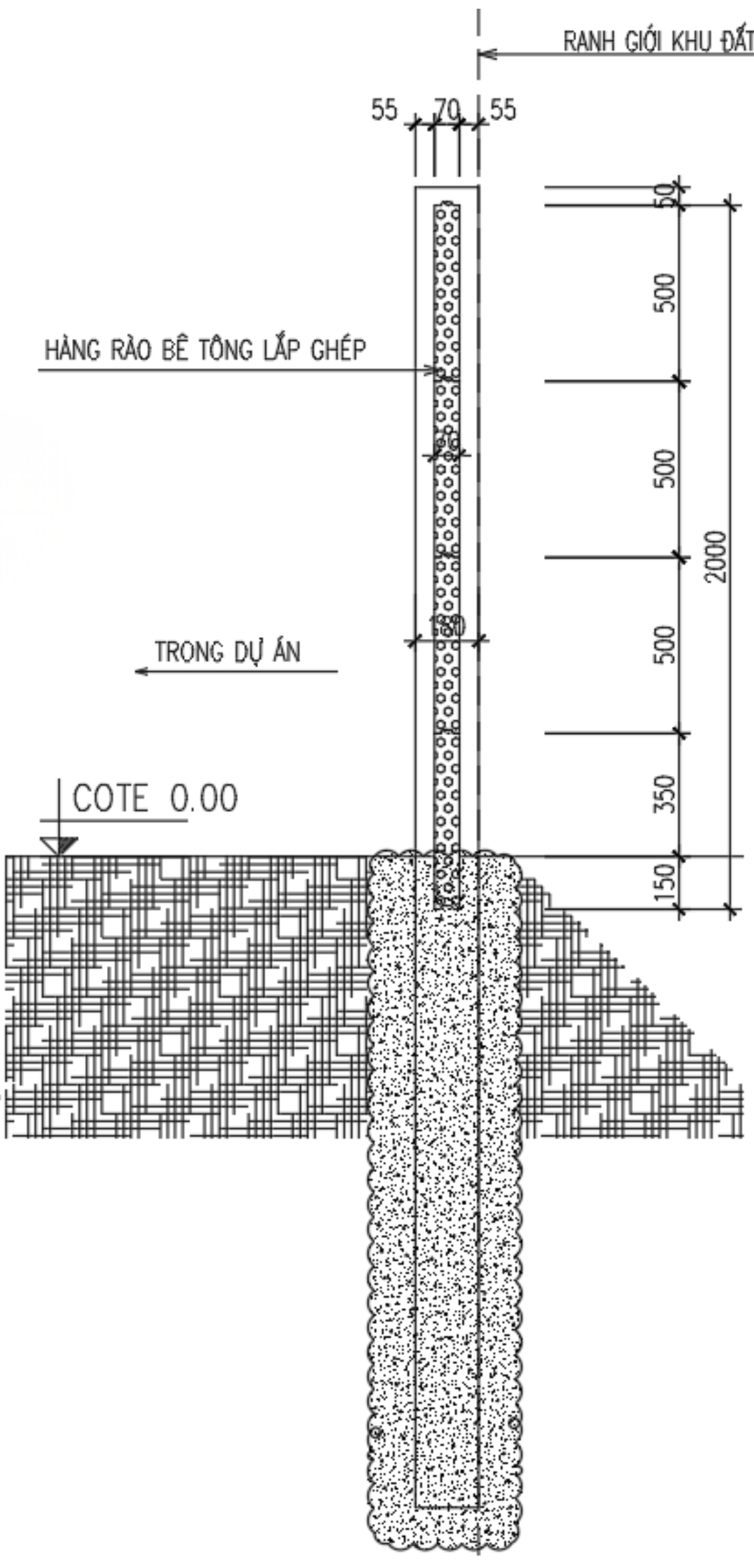
MẶT CẮT 1 - 1
